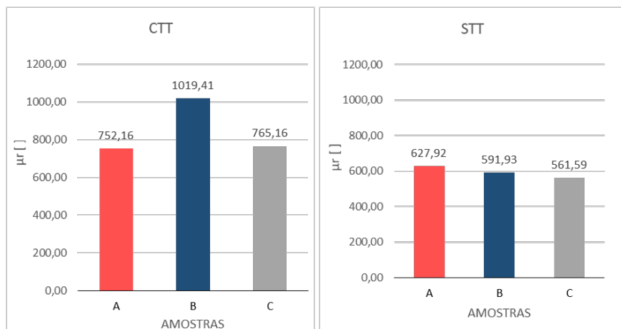
Figura 9 - Permeabilidade Magnética.
